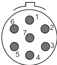
M12插座引脚图
